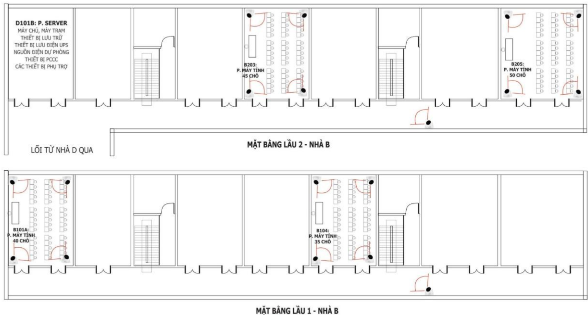
SƠ ĐỒ 2 : MẶT BẰNG TỔ CHỨC THI TRÊN MÁY TÍNH (LẦU 1, LẦU 2 NHÀ B - CƠ SỞ ĐÌNH TIỀN HOÀNG)
