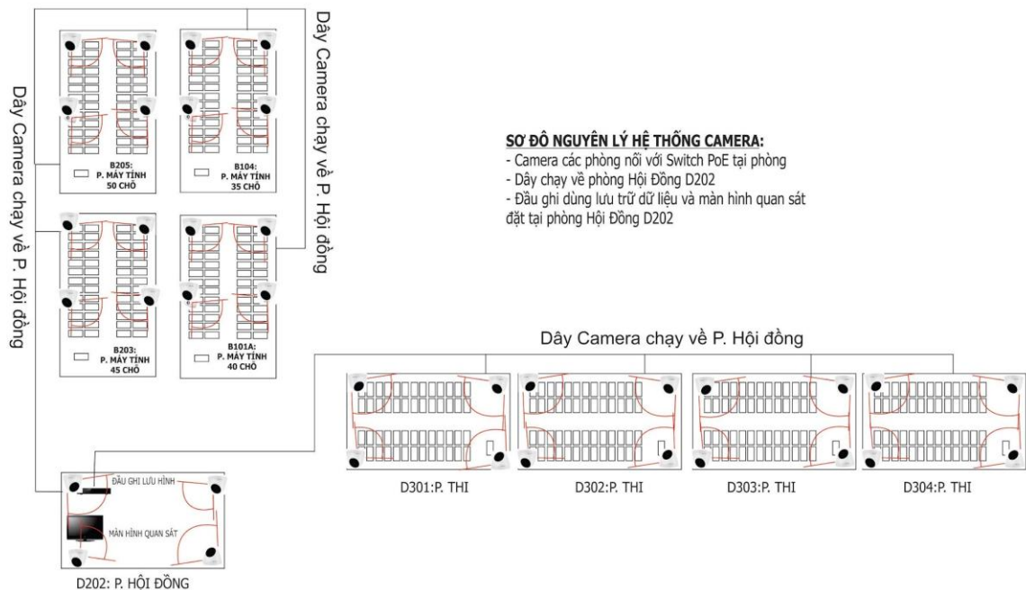
SƠ ĐỒ 4: MẶT BẰNG LẮP ĐẶT HỆ THỐNG CAMERA GIÁM SÁT TẠI CÁC PHÒNG THI
